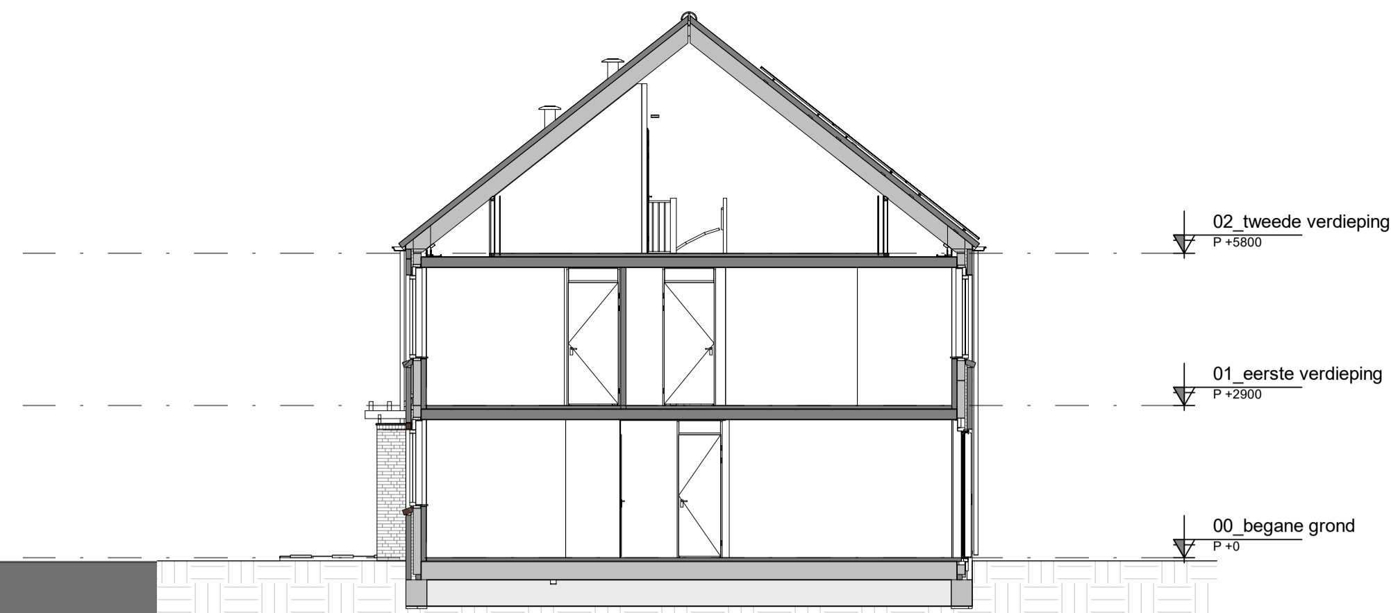
Doorsnede A1
