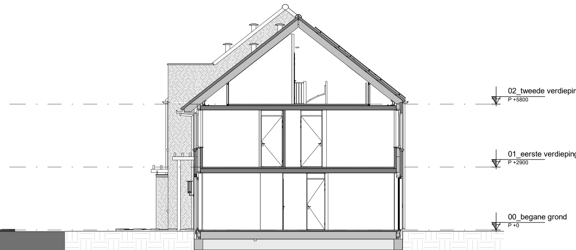
Doorsnede A2
