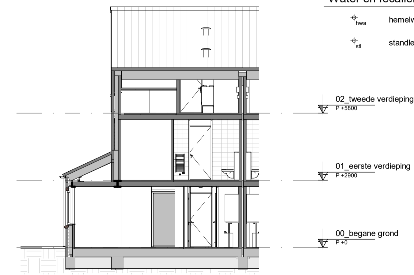
Doorsnede B
