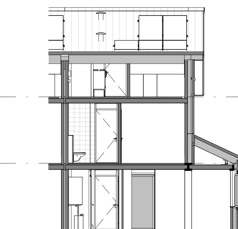
Doorsnede B
