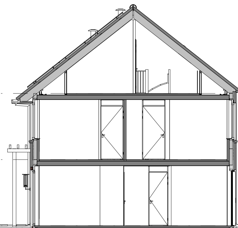
Doorsnede A
