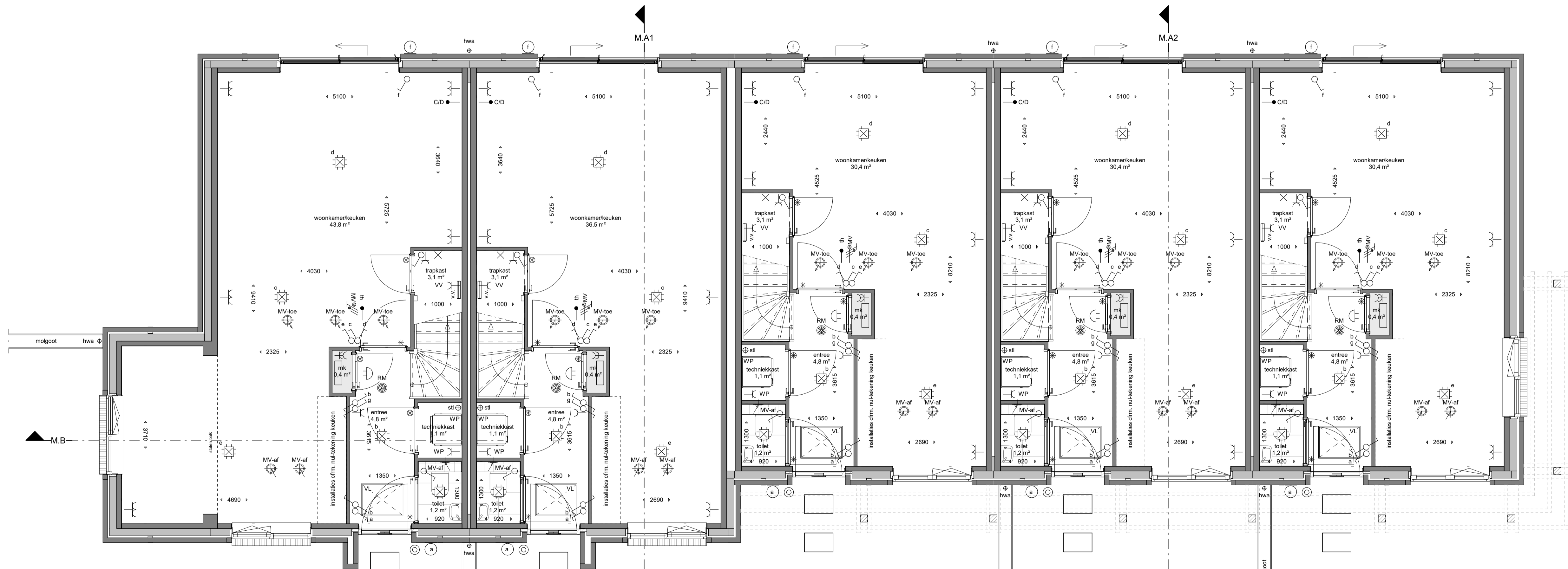
Begane Grond
