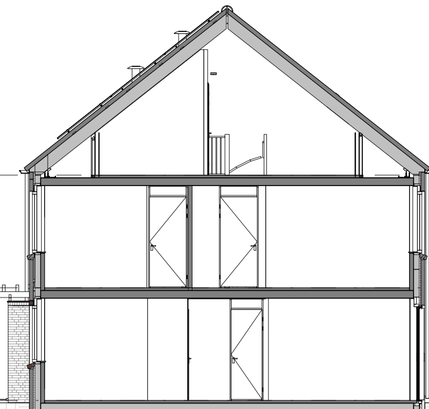
Doorsnede A1
