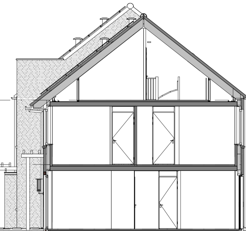
Doorsnede A2
