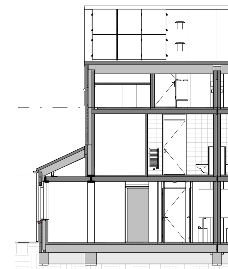
Doorsnede B
