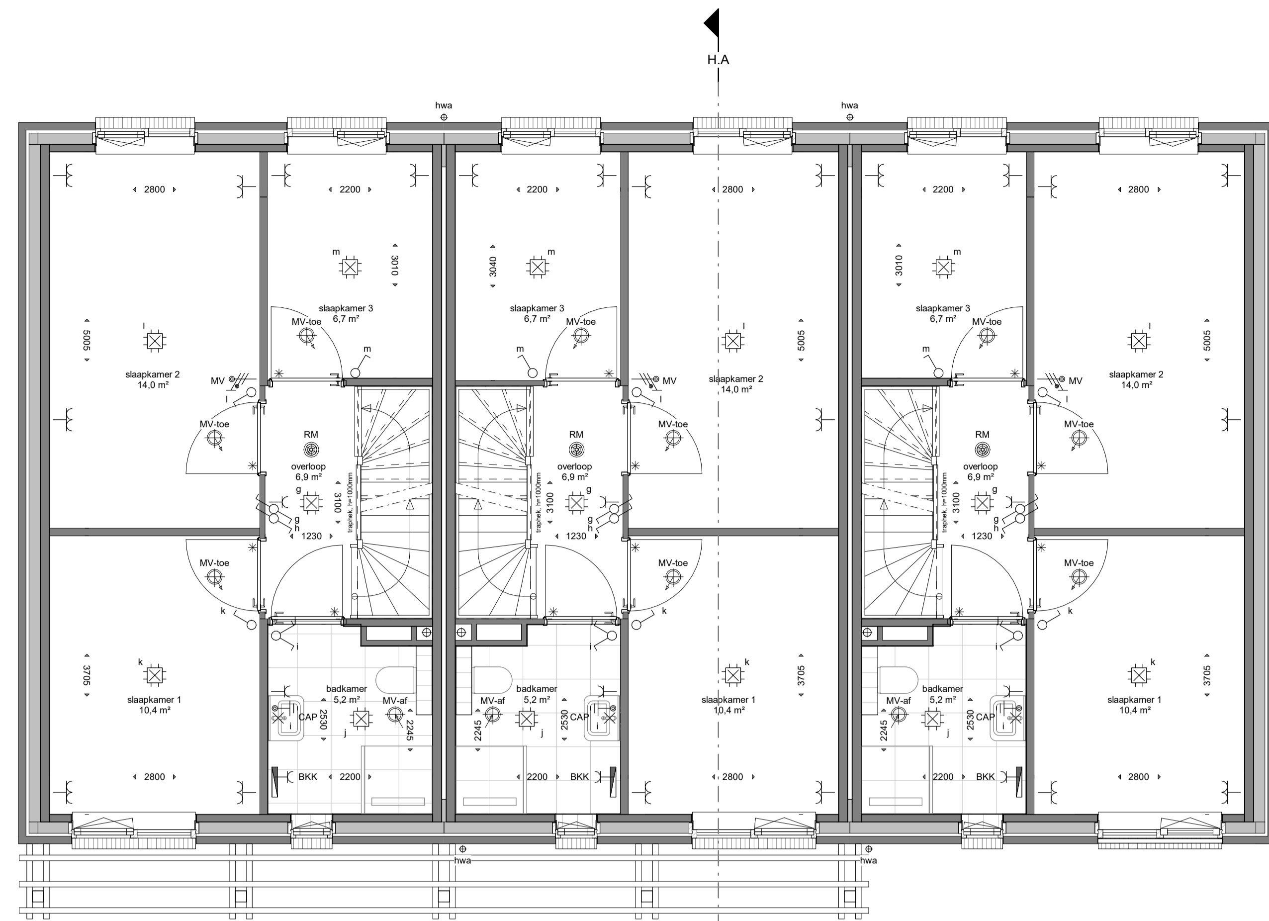
1e Verdieping Schaal 1 : 50
