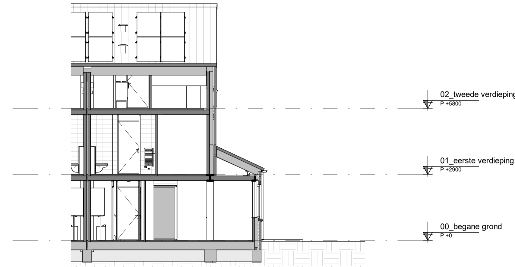
Doorsnede B
