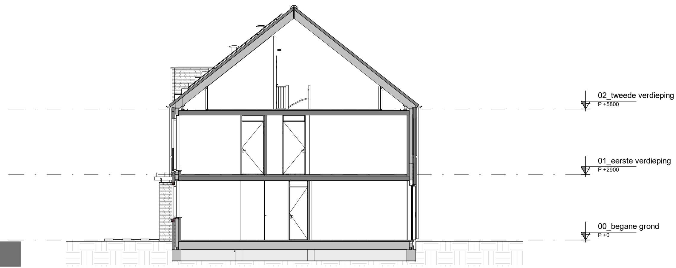
Doorsnede A
