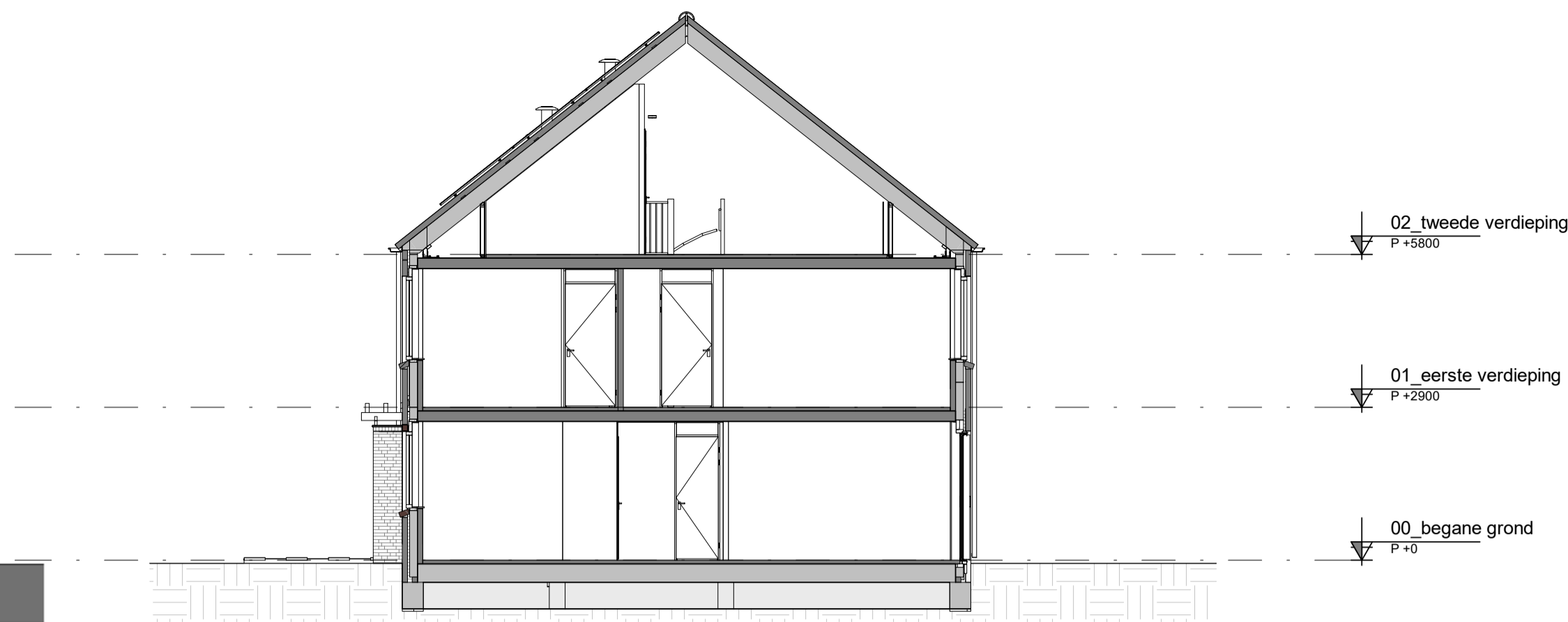
Doorsnede A
