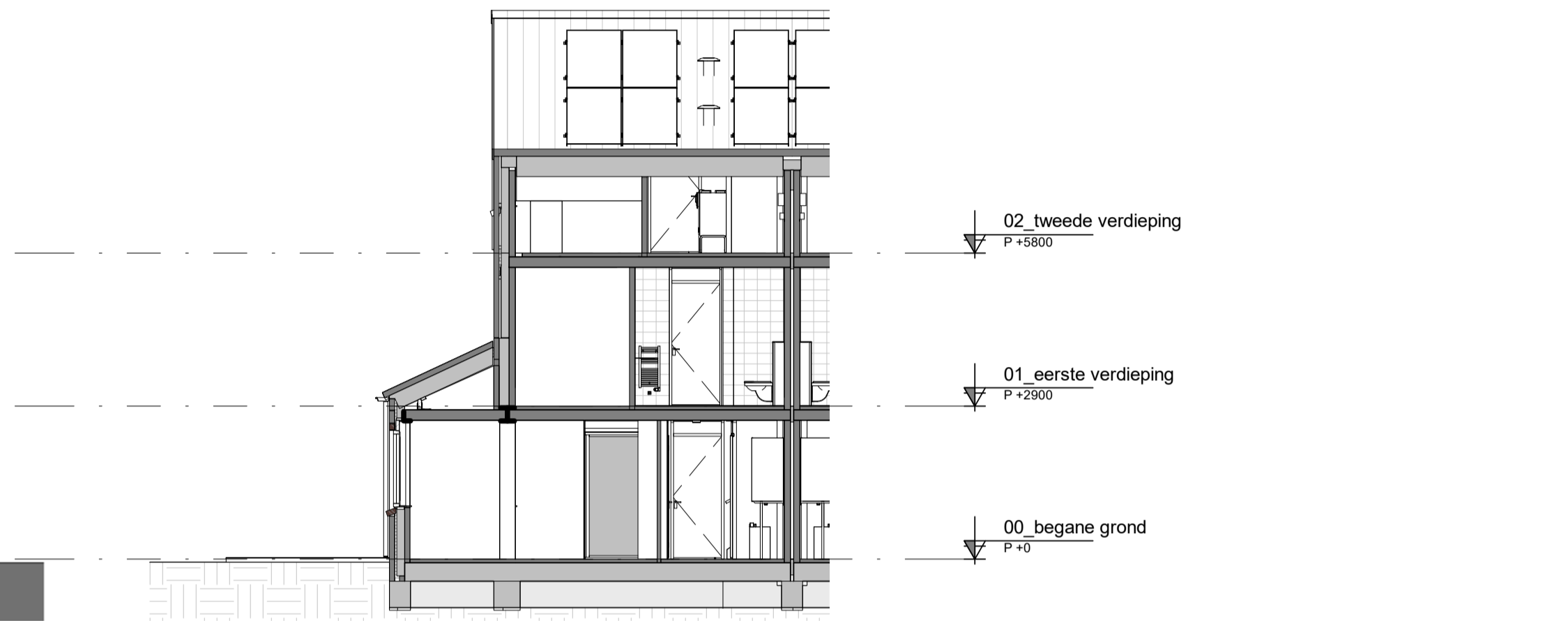
Doorsnede B
