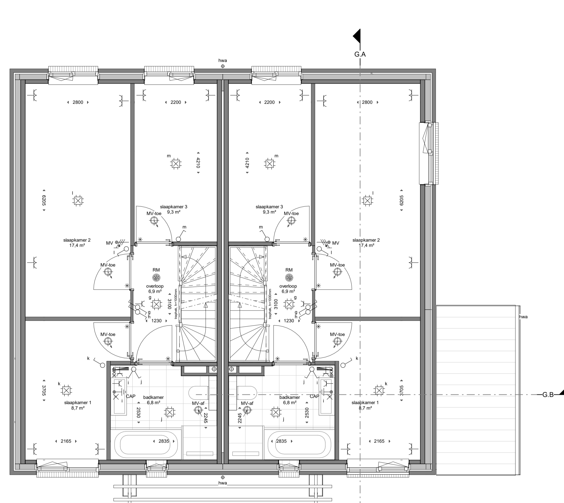
1e Verdieping Schaal 1:50
