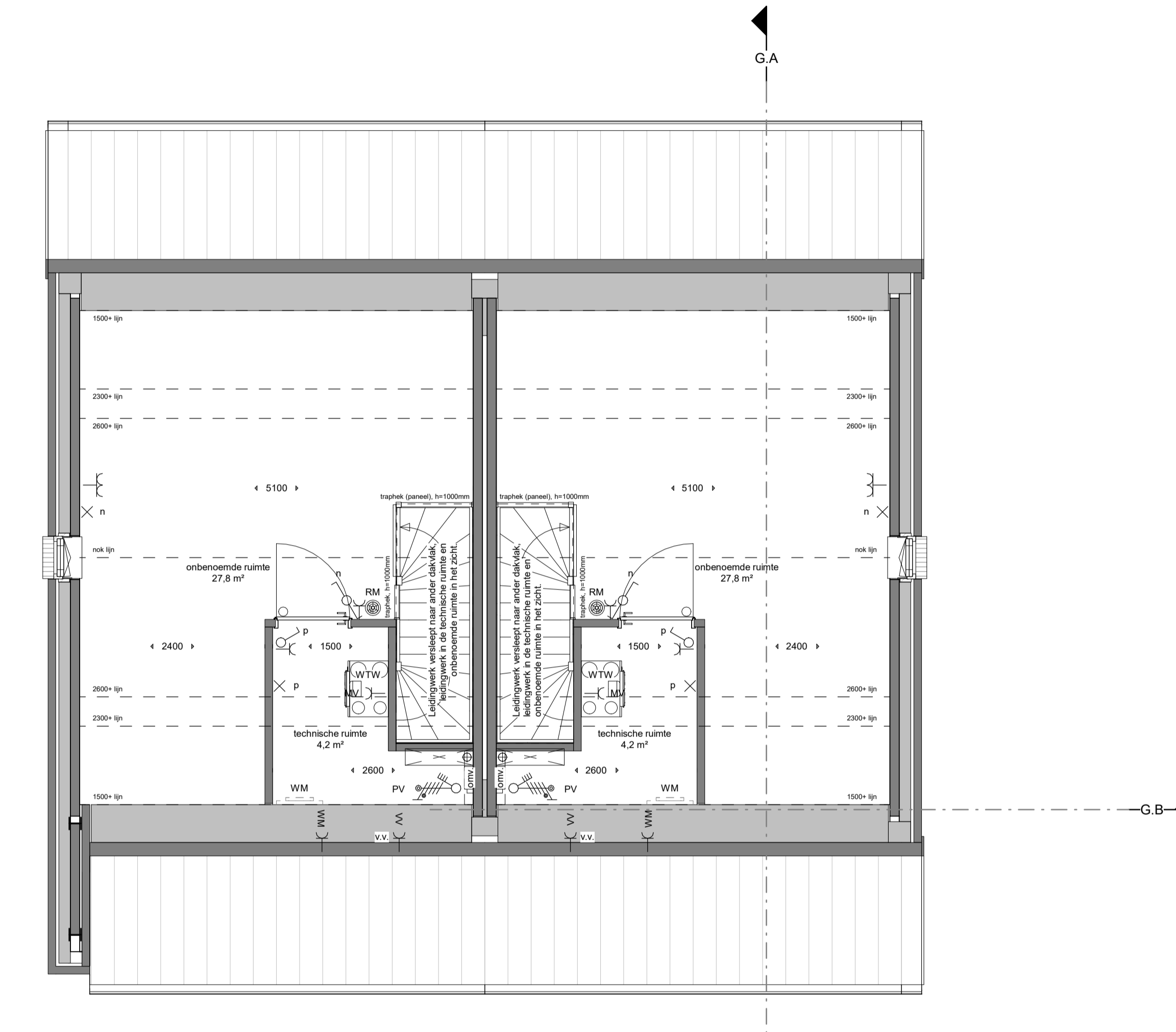
2e Verdieping Schaal 1:50
